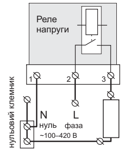
Схема 1. Спрощена внутрішня схема та схема підключення
