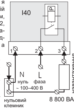
Схема 1. Спрощена внутрішня схема і схема підключення
